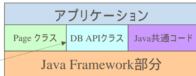
アプリケーションの静的構成
